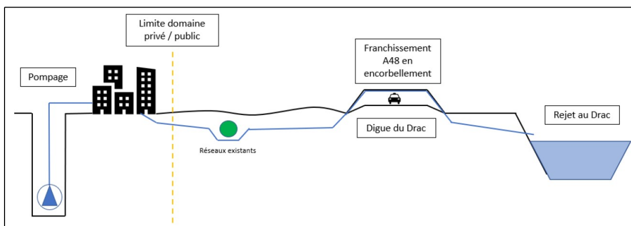
Figure 2: Schéma de principe du réseau d'exhaure (source : résumé non-technique des travaux).
